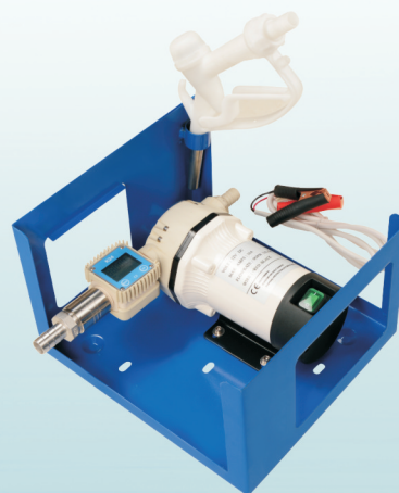
移动组合尿素泵 USN-WUP12
